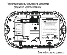
Рисунок 4. Светильника CA-7008Б. Вид сзади
