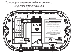
Рисунок 4. Светильник 75-009-IP30-SENSOR-EM. Вид сзади
