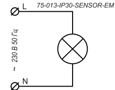
Рисунок 6 - Схема подключения светильника 75-013-IP30-SENSOR-EM
